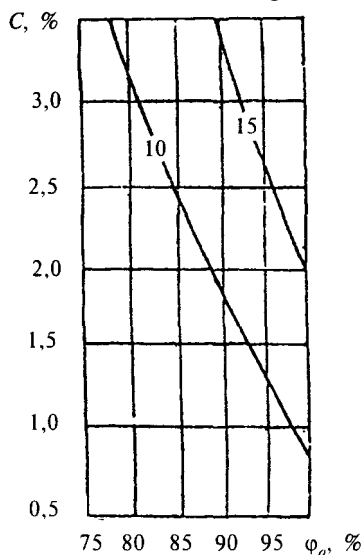
Рисунок Ц.3 — Изолинии сорбционного влагосодержания керамзитобетона \rho_0 = 1200 кг/м 3 , содержащего хлорид магния, при изменении относительной влажности воздуха \varphi_a , %, и массового солесодержания C , %
