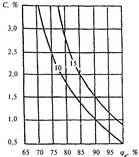
Рисунок Ц.1 — Изолинии сорбционного влагосодержания керамзитобетона \rho_0 = 1200 кг/м 3 , содержащего хлорид натрия, при изменении относительной влажности воздуха \varphi_a , %, и массового солесодержания C , %
