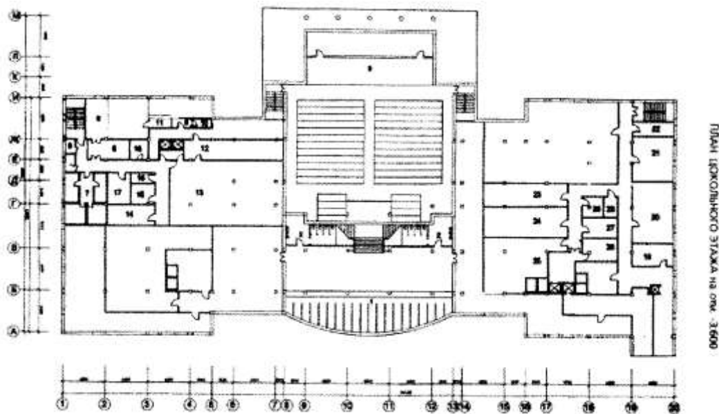
Рисунок Я.2 — План цокольного этажа
