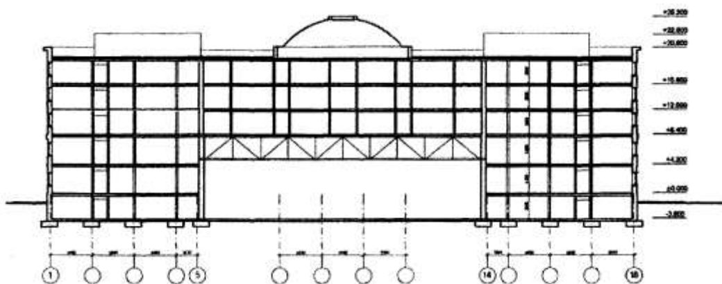
Рисунок Я.3 — Продольный разрез
