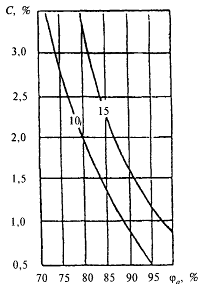
Рисунок Ц.4 — Изолинии сорбционного влагосодержания керамзитобетона \rho_0 = 1200 кг/м 3 , содержащего NaCl - 60 %, KCl - 30 %, MgCl 2 - 10 %, при изменении относительной влажности воздуха \varphi_a , %, и массового солесодержания C , %, в стенах флотофабрик
