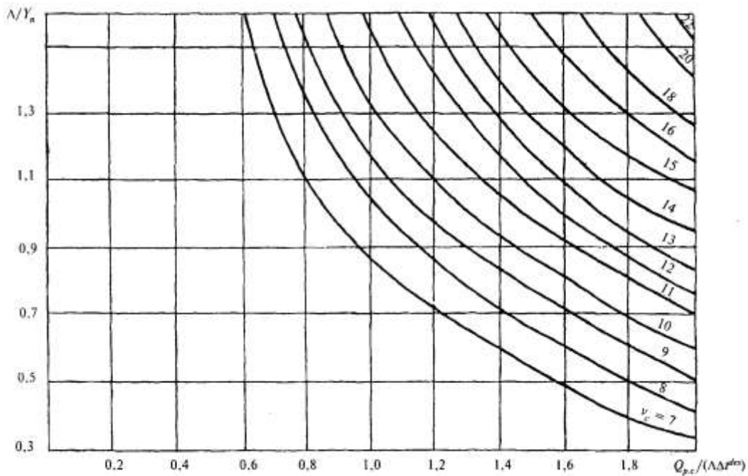
Рисунок 4 — График для подбора теплоаккумулирующих приборов (продолжительность зарядки 6 + 2 ч дневной подразрядки)
