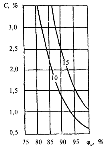
Рисунок Ц.2 — Изолинии сорбционного влагосодержания керамзитобетона \rho_0 = 1200 кг/м 3 , содержащего хлорид калия, при изменении относительной влажности воздуха \varphi_a , %, и массового солесодержания C , %
